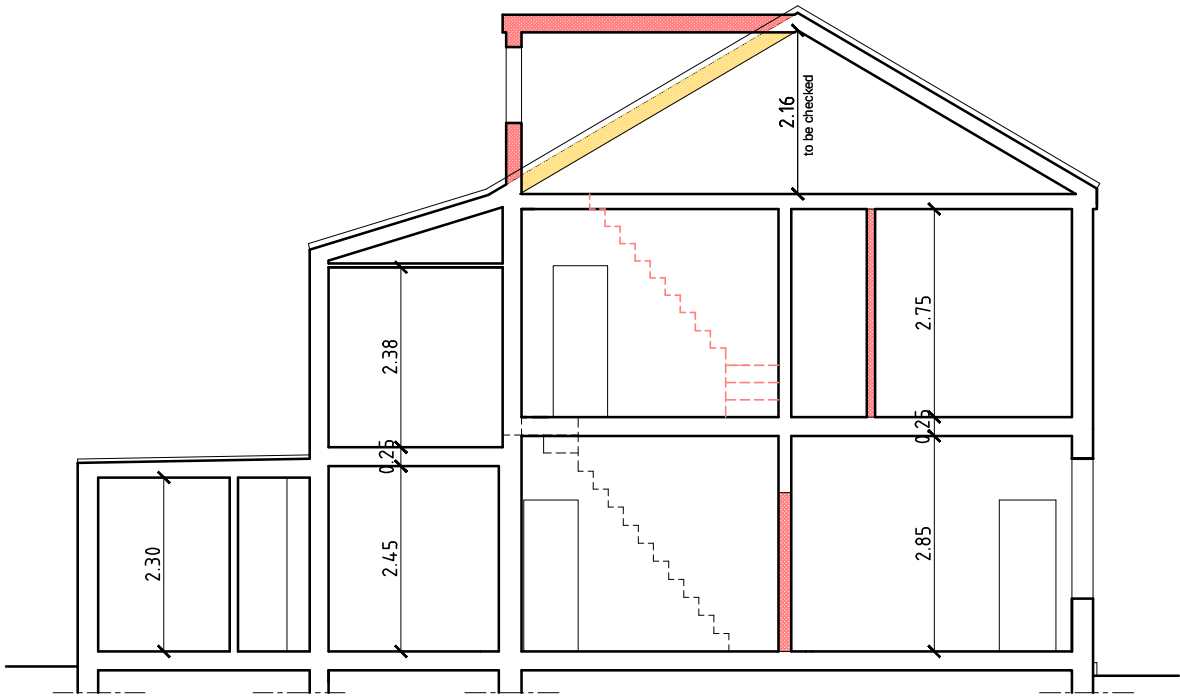
SECTION A-A
